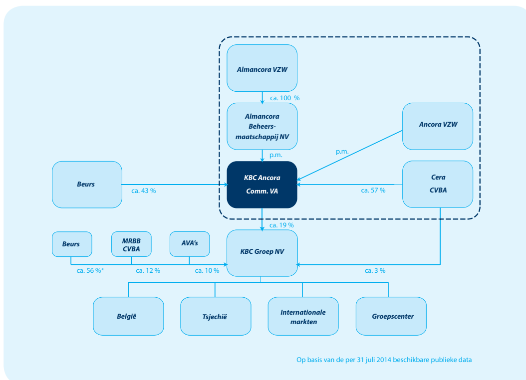
Grafiek 6: Groepsstructuur 7
