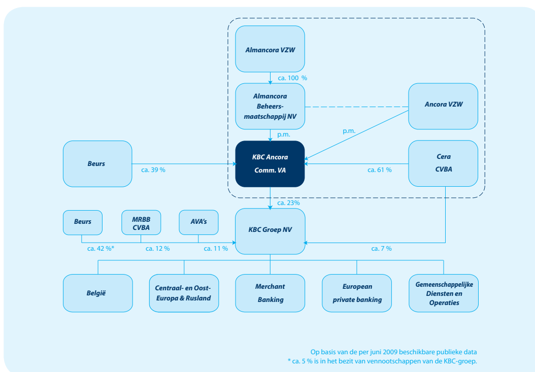
Grafiek 7: Groepsstructuur 6
